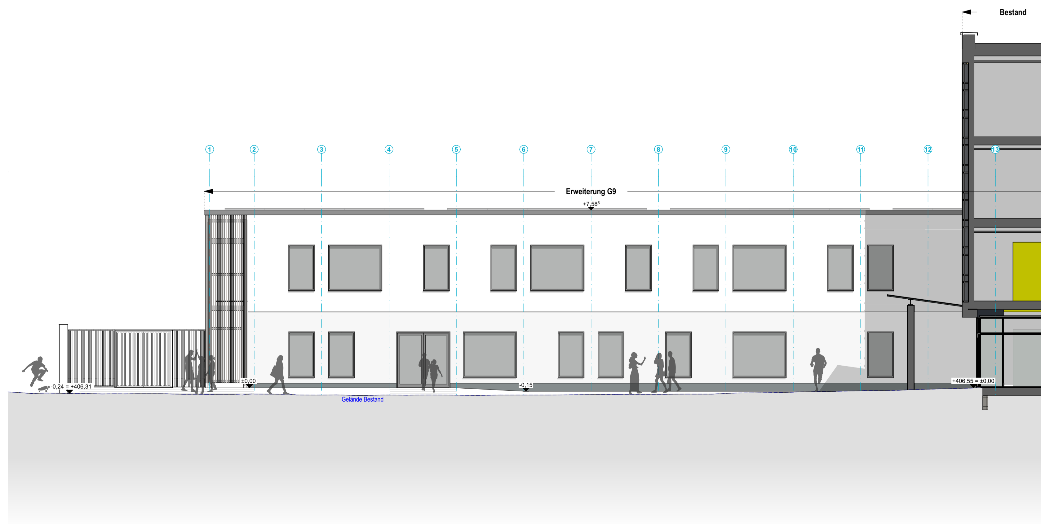
Ansicht Süd
