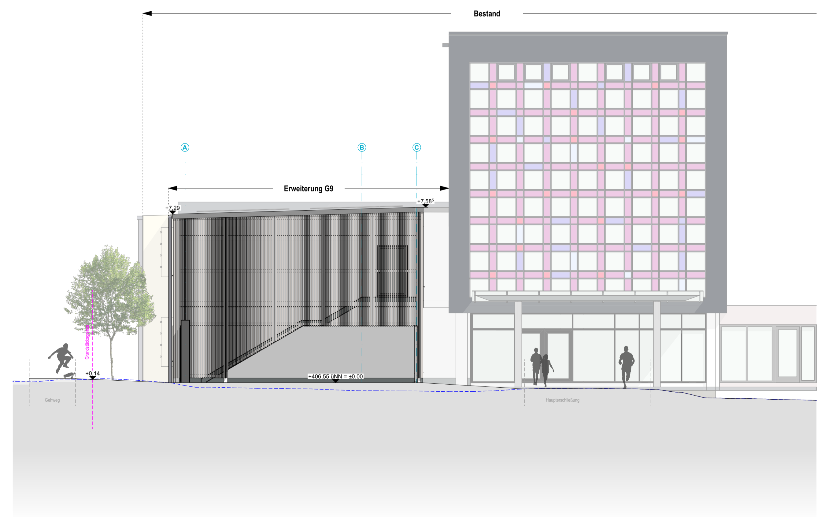
Ansicht Ost
